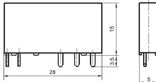
Rozměry relé v mm:
